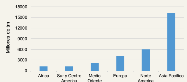
Emisiones globales de CO 2 por regiones al 2018
